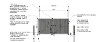
06 DUMPSTER ENCLOSURE ELEVATION Scale: 1:10
